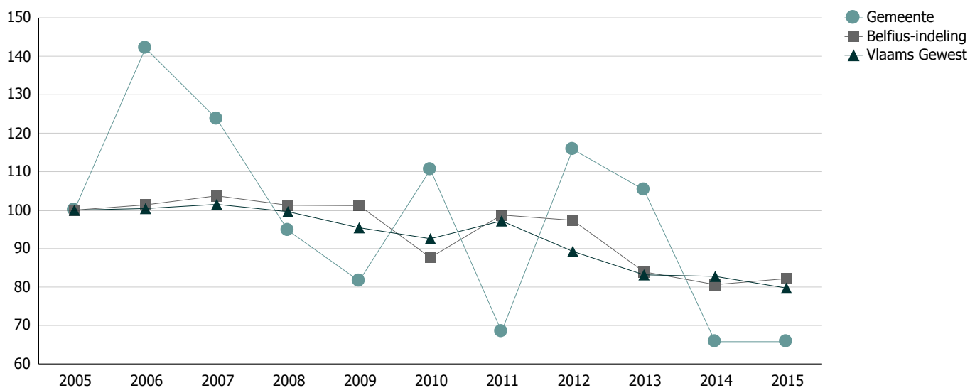
Evolutie verkeersongevallen (2005=100)
