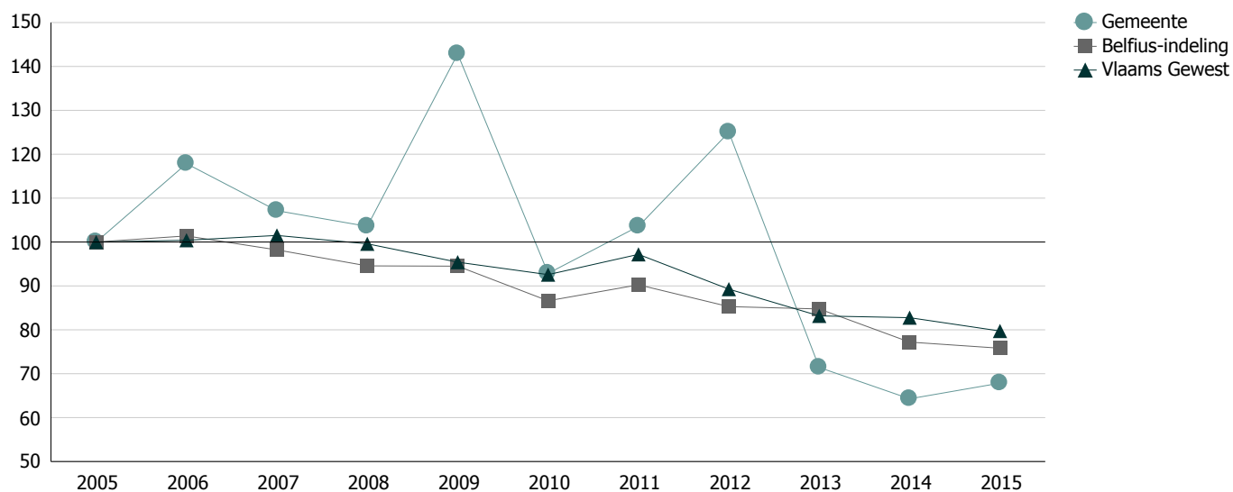
Evolutie verkeersongevallen (2005=100)
